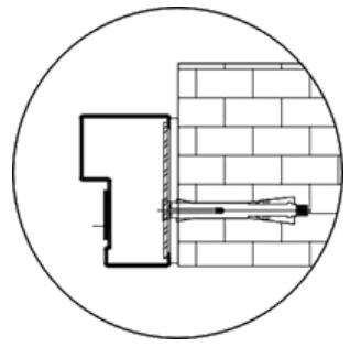
DETALLE A
